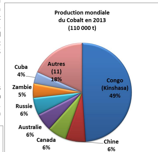
Figure6 : Production mondiale cobalt 2013, total de 110 000 tonnes métriques (Données tirées de l'USGS 2013).
