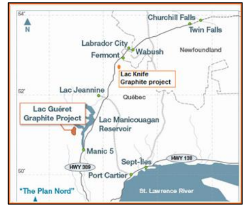
Figure 2 : Localisation des dépôts du Lac Guéret et du Lac Knife. (Modifiée de Mason Graphite, 2013).
