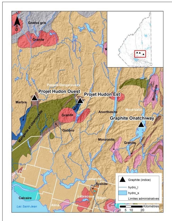
Figure 3: Localisation des indices de graphite ((SIGÉOM, 2015 et CRRNT, 2011 / carte géologique : Intégration CONSOREM 2016, modifiée de SIGÉOM 2015 et de CERM-PACES 2013). Carte géologique en ligne à www.crm-slsj.ca .
